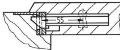
Profil einer Falztür
